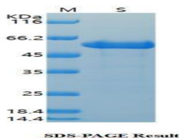
SDS-PAGE Result
